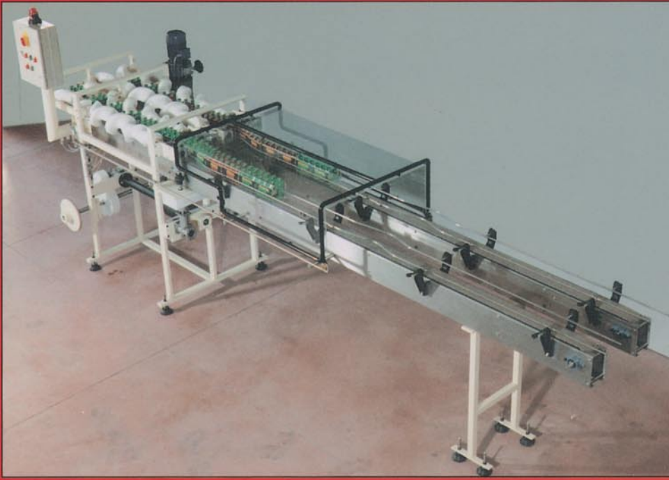
Gruppo rotatore cluster. Cluster rotator. Groupe rotateur cluster.
