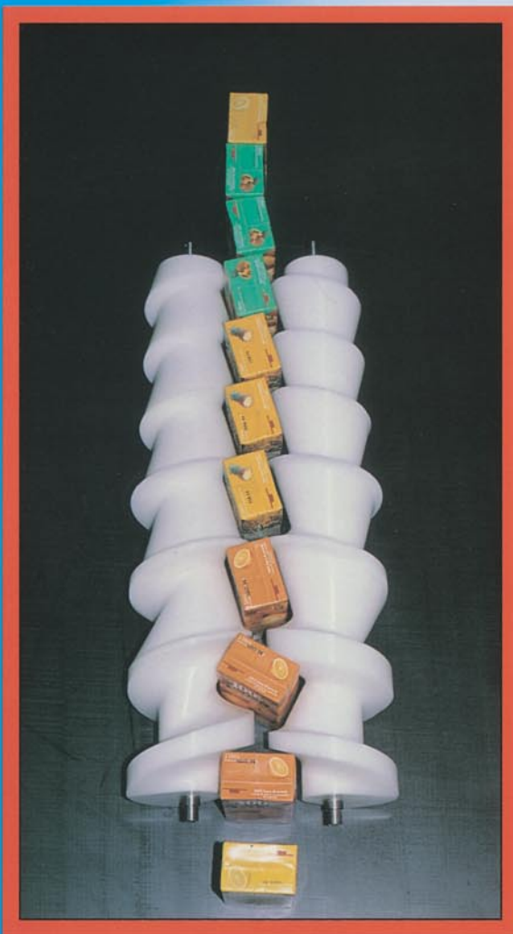
Rotatori per ogni tipo di contenitore. Rotators for any kind of containers. Rotateurs pour tous les genres de boites.
